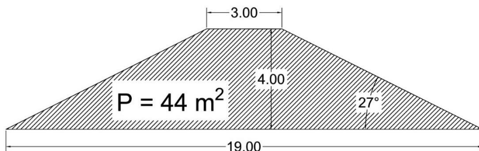
Slika 1: Poprečni presek pregradnog bedema
