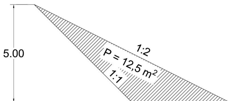
Slika 2: Proračunski presek kod ublažavanja pada obodnih kosina
